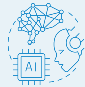
Generative AI
